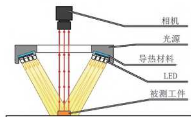
环形光源打光示意图
