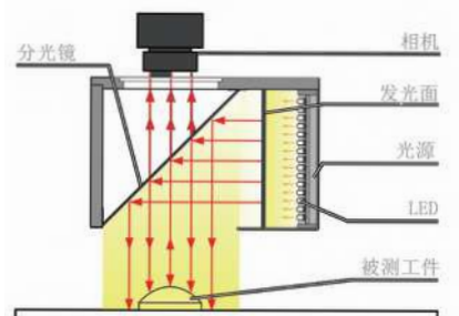
同轴光源打光示意图
